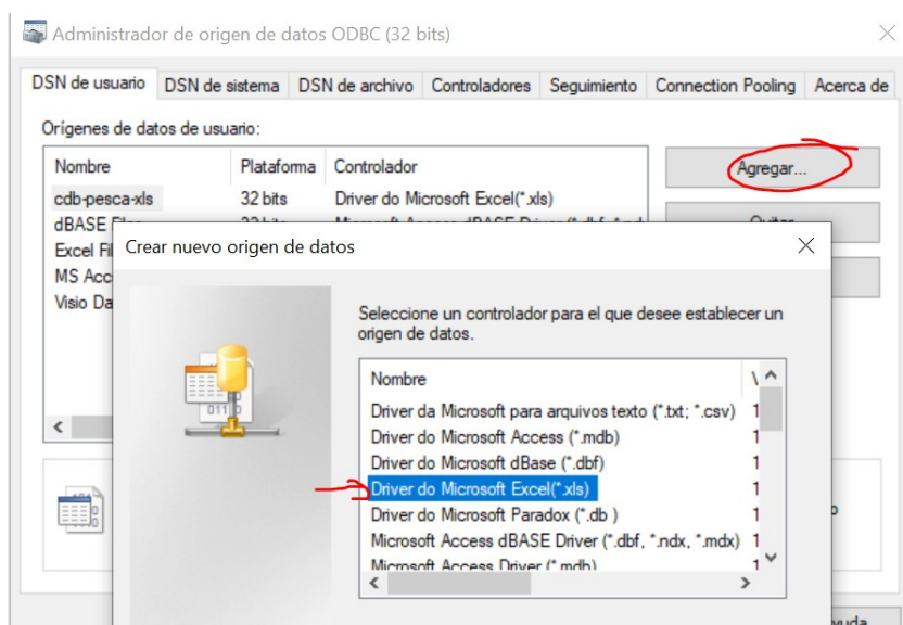
Figura 4. Agregar un origen de datos con el controlador de Excel (*.xls)
